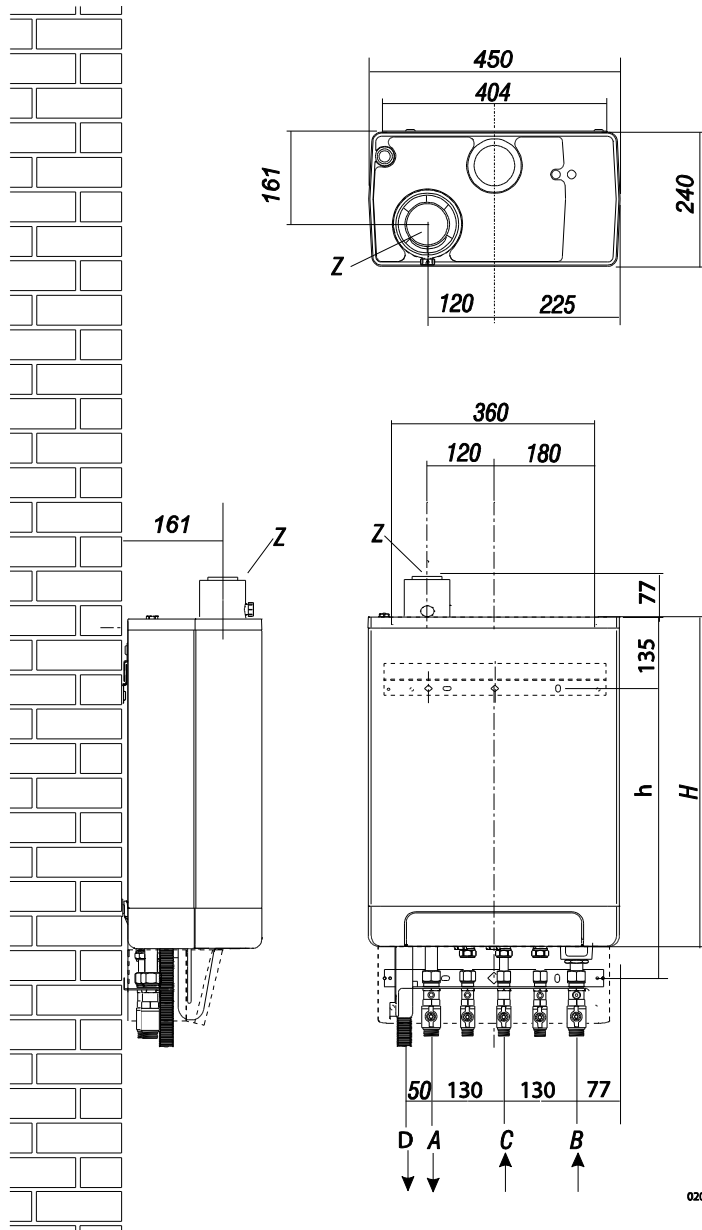
Toestel + montagebeugel
