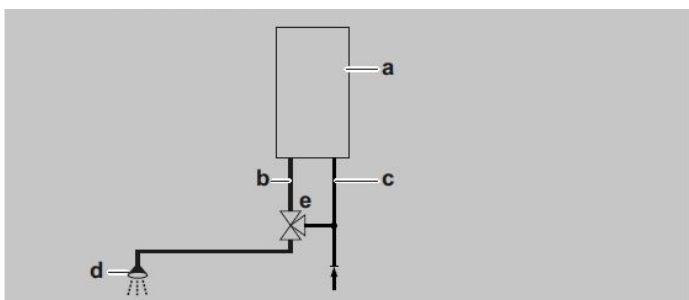
a= kocioł, b= CWU z kotła, c= wlot zimnej wody, d= prysznic, e= zawór termostaticzny (nie należy do wyposażenia)
